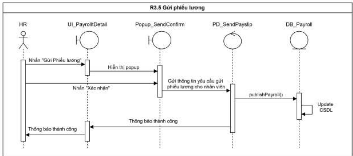
Hình 3.23 Biểu đồ tuần tự “Gửi phiếu lương”
