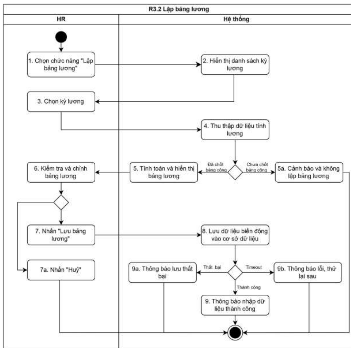
Hình 3.40 Biểu đồ hoạt động “Lập bảng lương”
