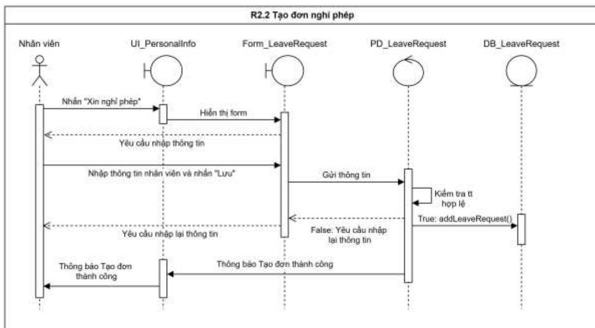
Hình 3.14 Biểu đồ tuần tự “Tạo đơn nghỉ phép”
