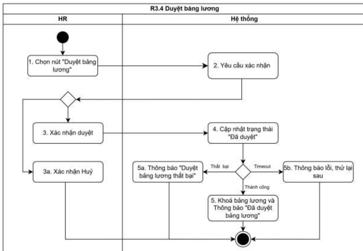
Hình 3.42 Biểu đồ hoạt động “Duyệt bảng lương”
