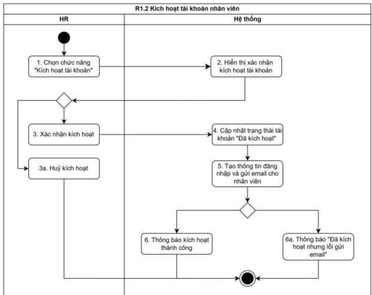
Hình 3.28 Biểu đồ hoạt động “Kích hoạt tài khoản nhân viên”
