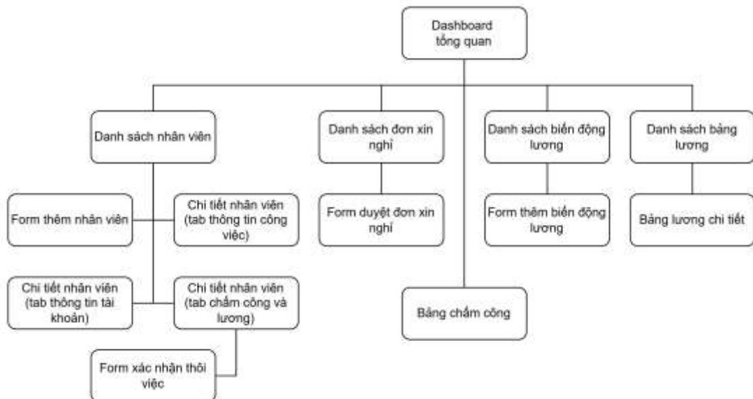
Hình 3.51 Lược đồ di chuyển tổng thể cho HR
