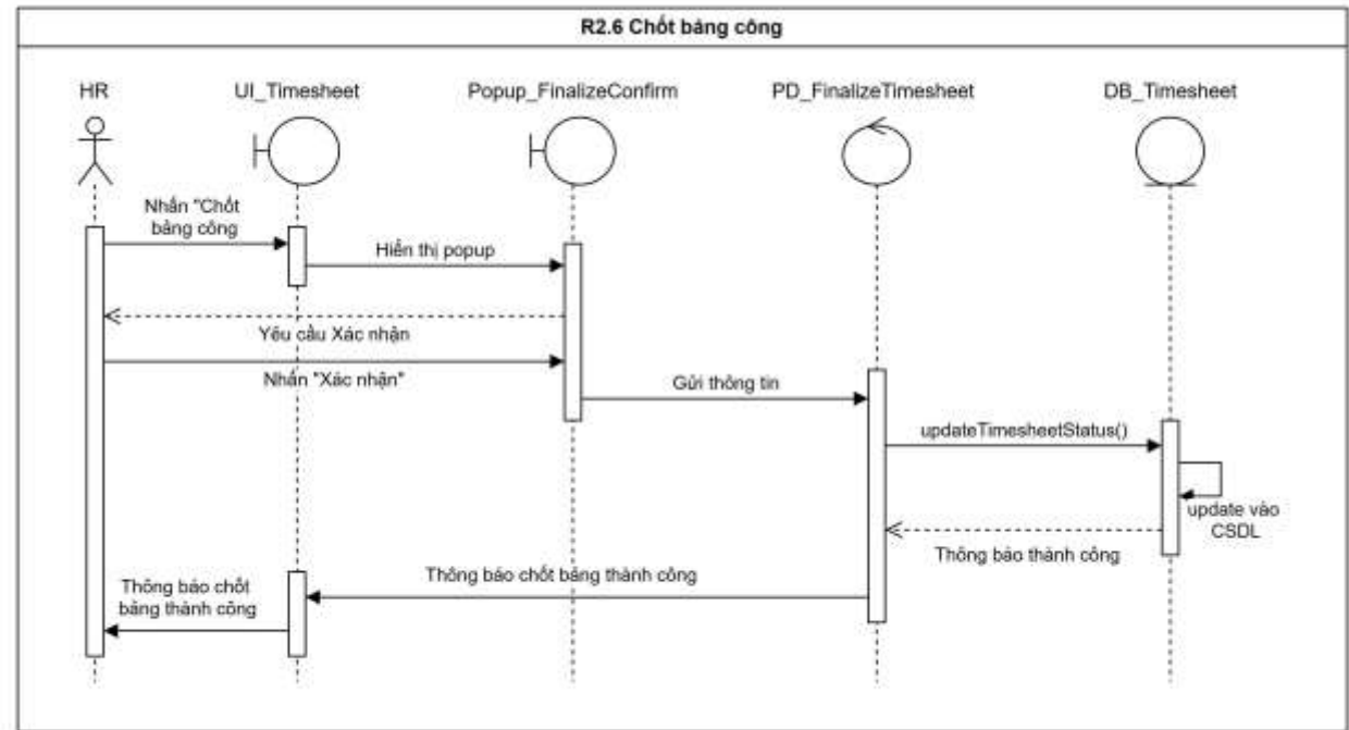
Hình 3.18 Biểu đồ tuần tự “Chốt bảng công”
