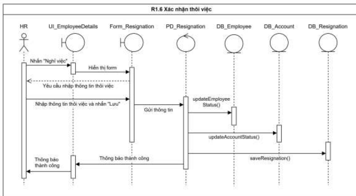
Hình 3.12 Biểu đồ tuần tự “Xác nhận thôi việc”
