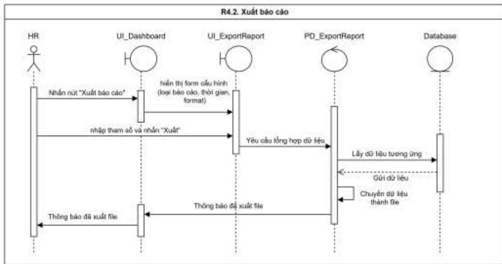
Hình 3.26 Biểu đồ tuần tự “Xuất báo cáo”
