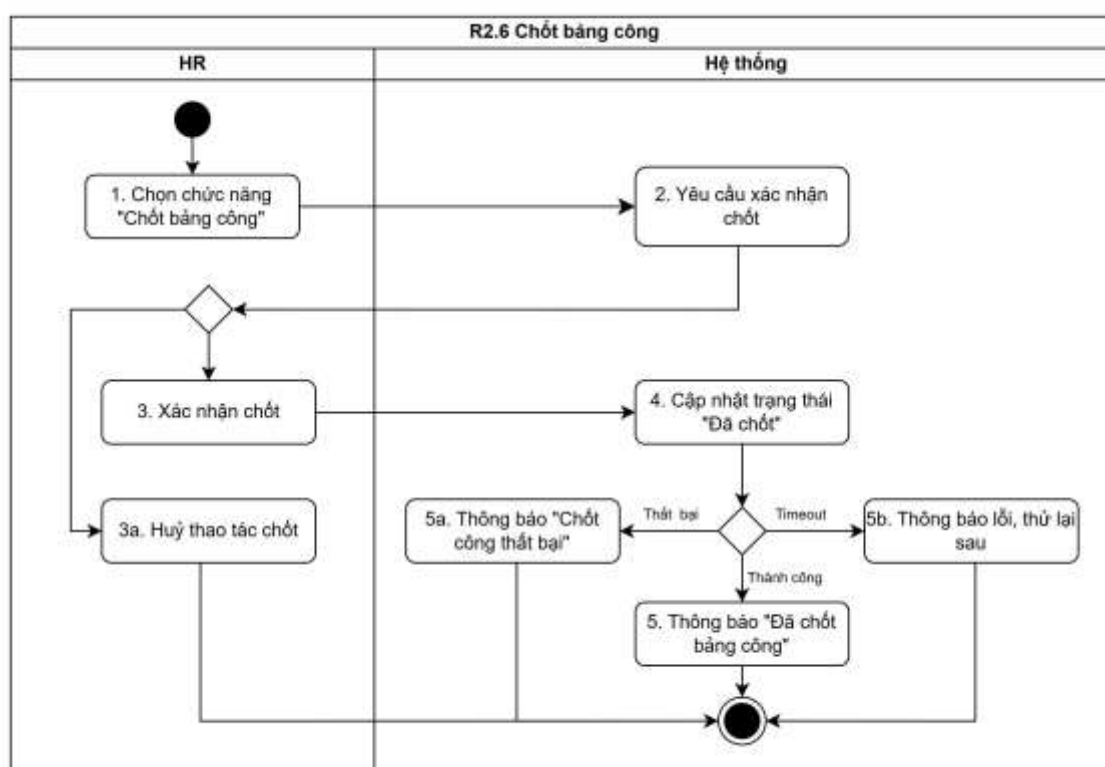
Hình 3.38 Biểu đồ hoạt động “Chốt bảng công”
