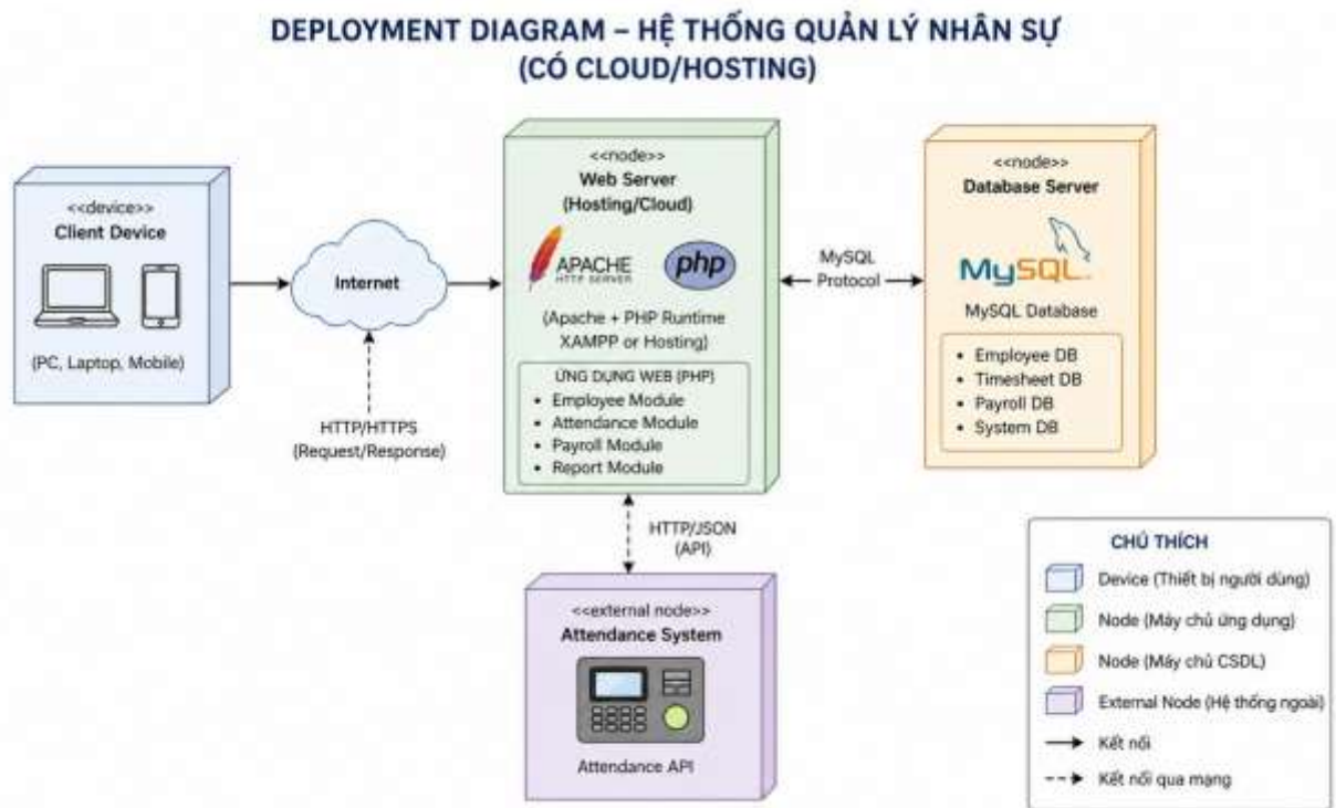
Hình 3.49 Biểu đồ triển khai
