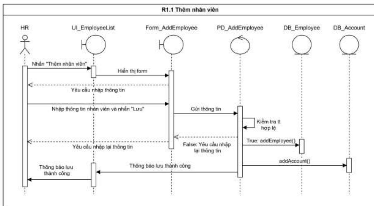
Hình 3.7 Biểu đồ tuần tự “Thêm nhân viên”
