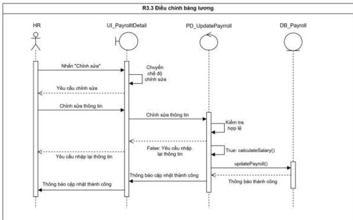
Hình 3.21 Biểu đồ tuần tự “Điều chỉnh bảng lương”
