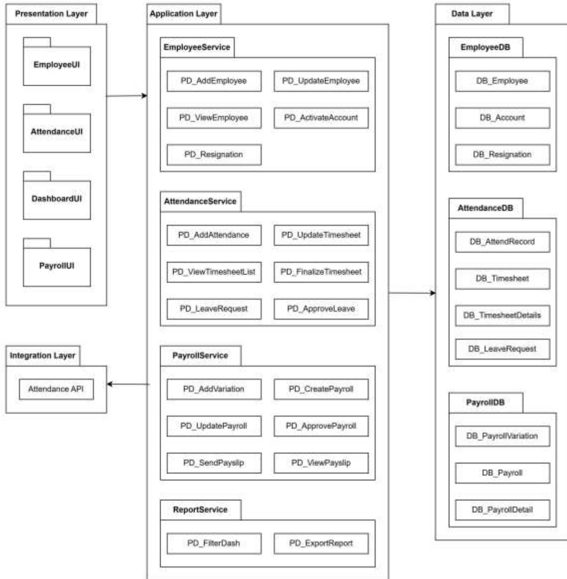
Hình 3.47 Biểu đồ gói
