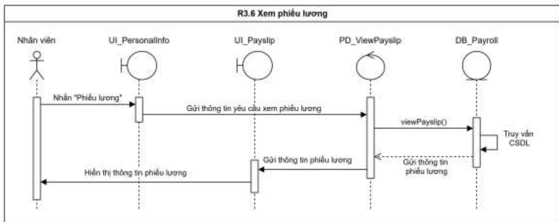
Hình 3.24 Biểu đồ tuần tự “Xem phiếu lương”
