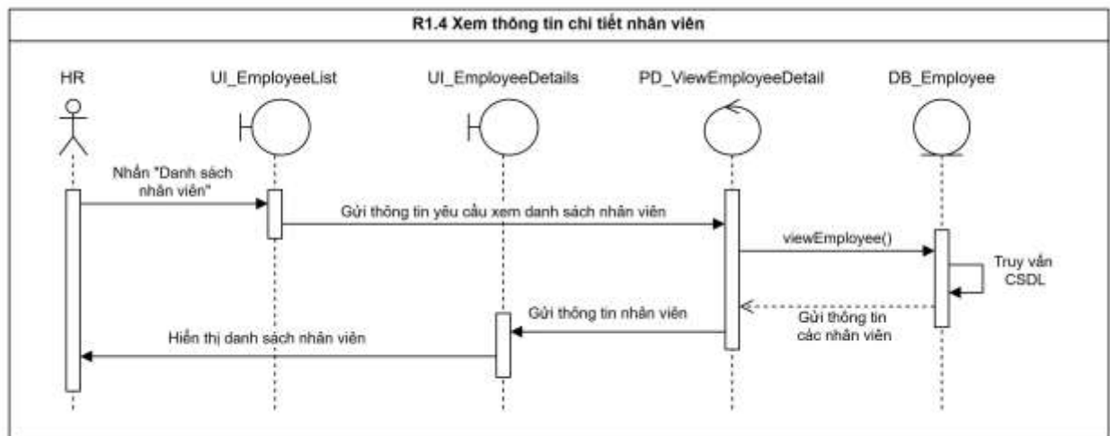
Hình 3.10 Biểu đồ tuần tự “Xem thông tin chi tiết nhân viên”
