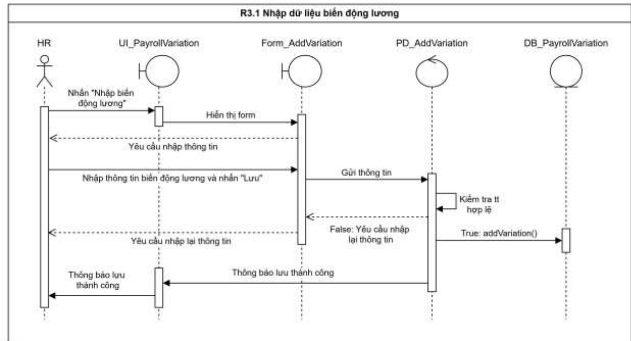
Hình 3.19 Biểu đồ tuần tự “Nhập dữ liệu biến động lương”
