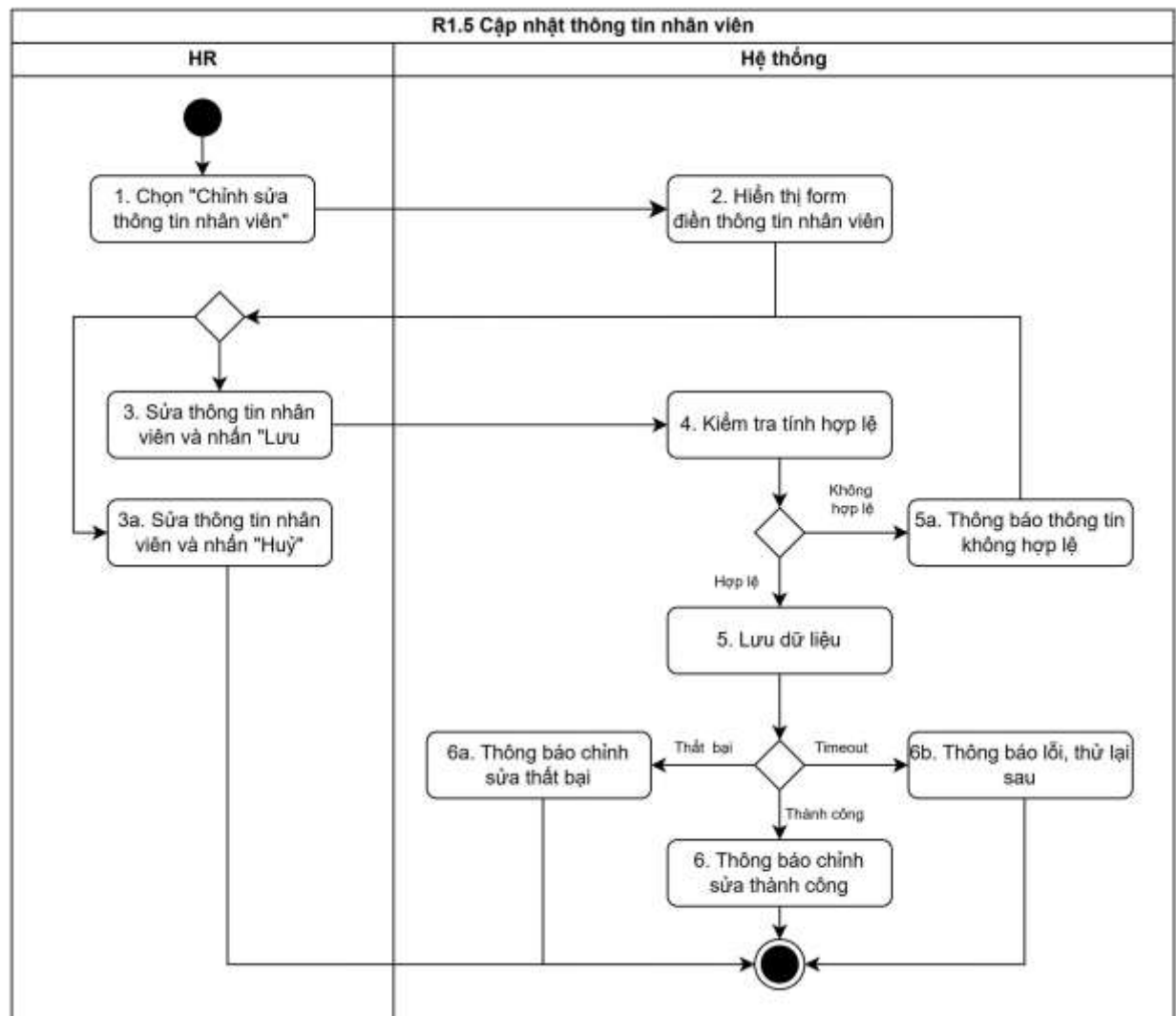
Hình 3.31 Biểu đồ hoạt động “Cập nhật thông tin nhân viên”
