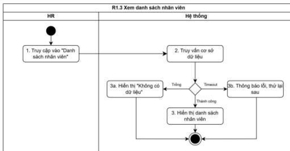
Hình 3.29 Biểu đồ hoạt động “Xem danh sách nhân viên”
