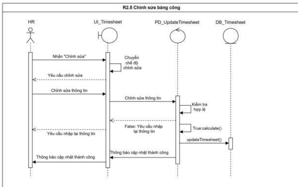
Hình 3.17 Biểu đồ tuần tự “Chỉnh sửa công”
