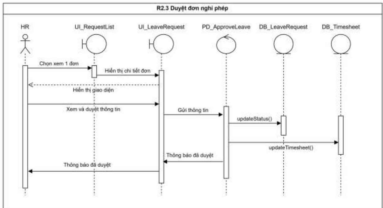
Hình 3.15 Biểu đồ tuần tự “Duyệt đơn nghỉ phép”
