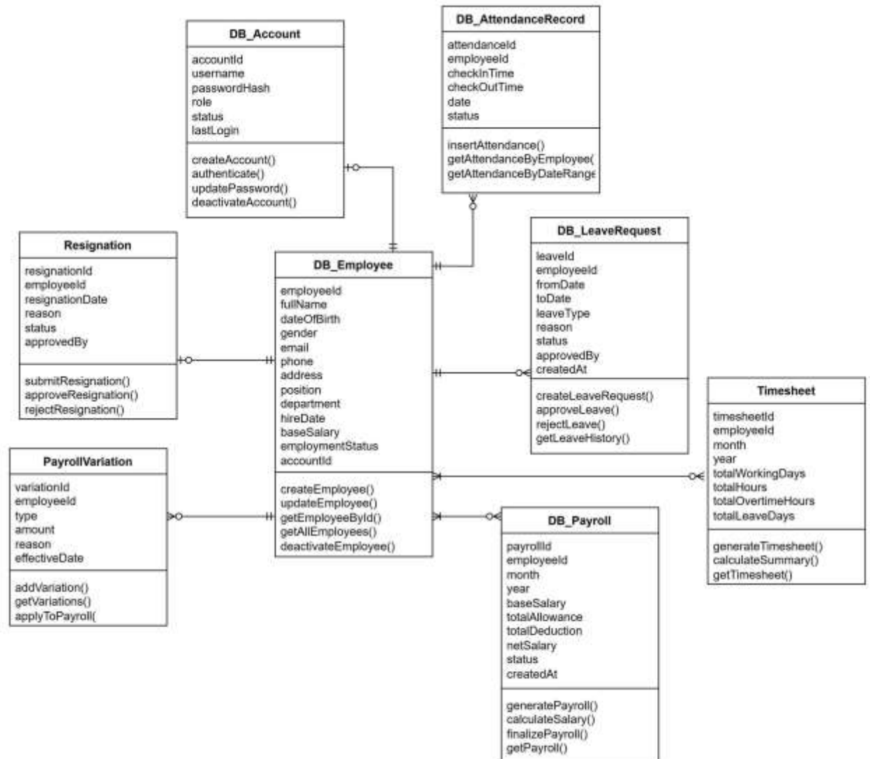
Hình 3.6 Biểu đồ lớp
