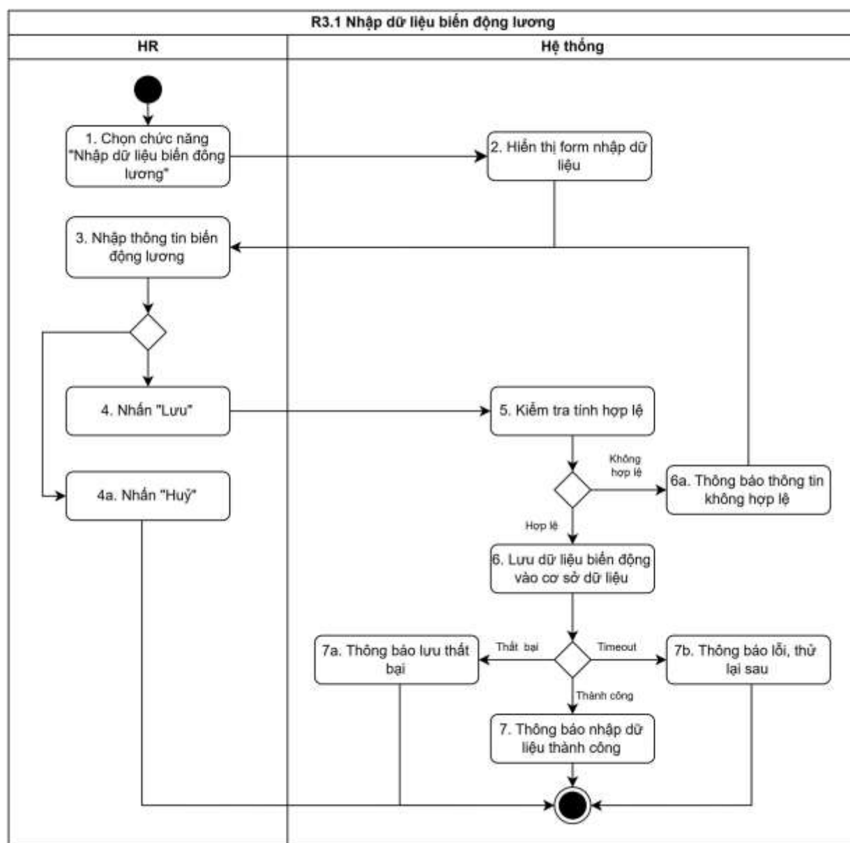
Hình 3.39 Biểu đồ hoạt động “Nhập dữ liệu biến động lương”
