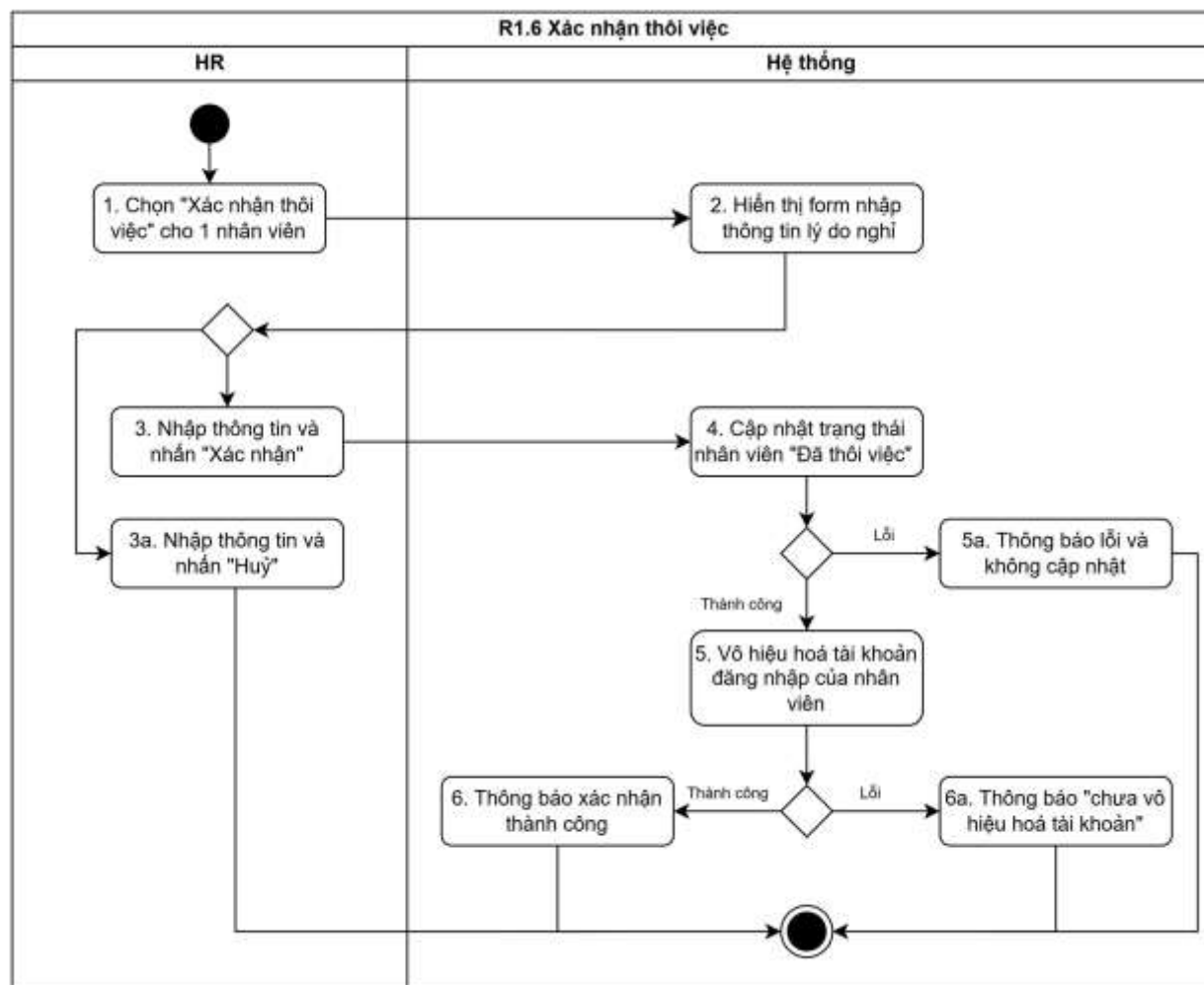
Hình 3.32 Biểu đồ hoạt động “Xác nhận thôi việc”
