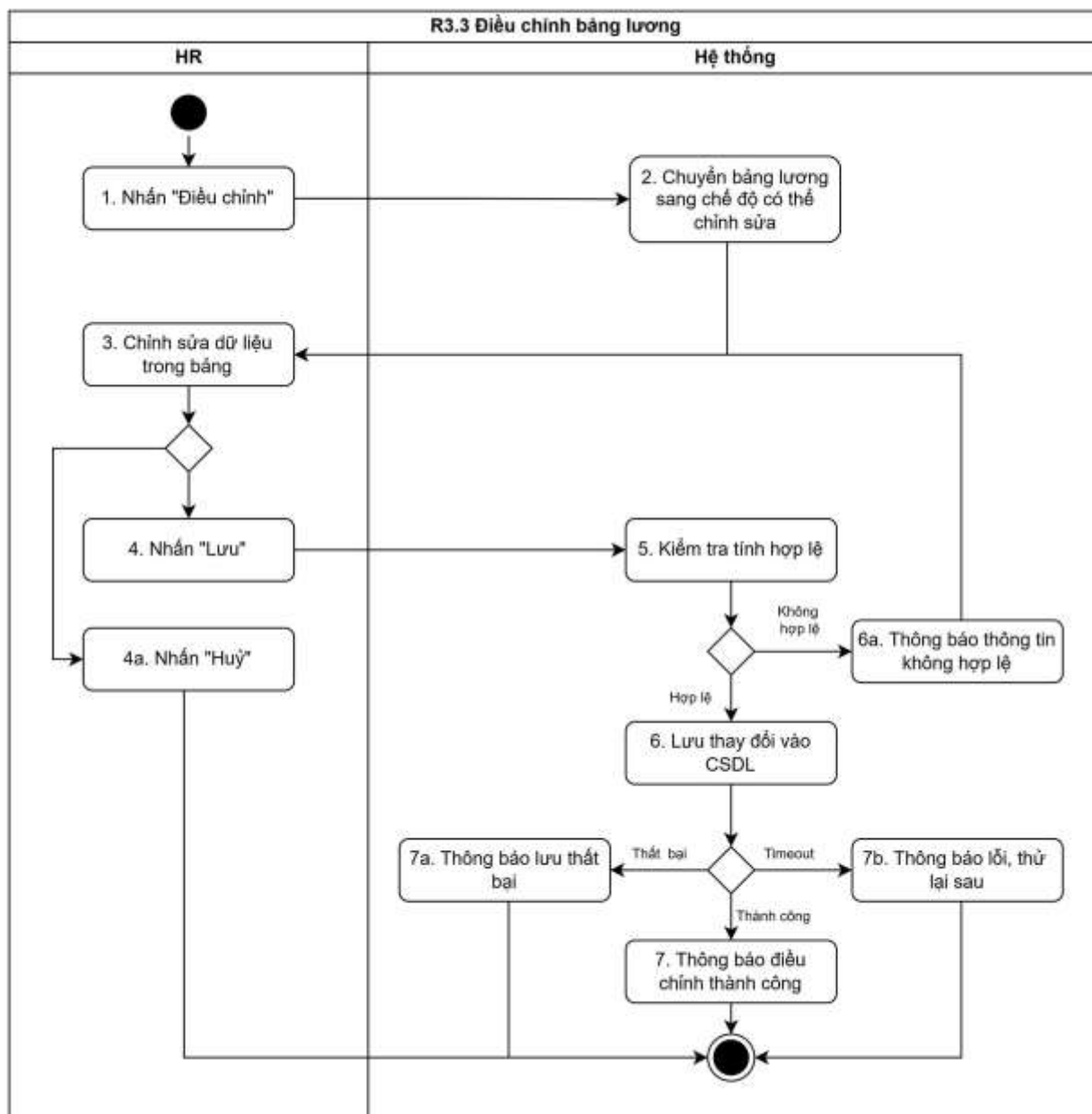
Hình 3.41 Biểu đồ hoạt động “Điều chỉnh bảng lương”
