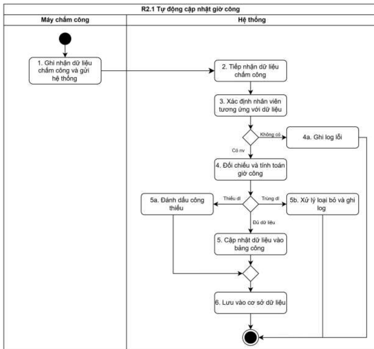
Hình 3.33 Biểu đồ hoạt động “Tự động cập nhật giờ công”
