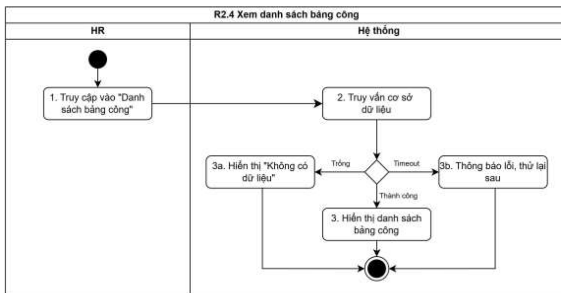
Hình 3.37 Biểu đồ hoạt động “Xem danh sách bảng công”
