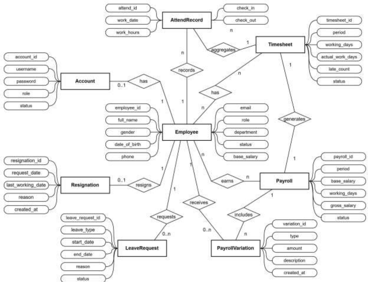
Hình 3.50 Lược đồ ERD
