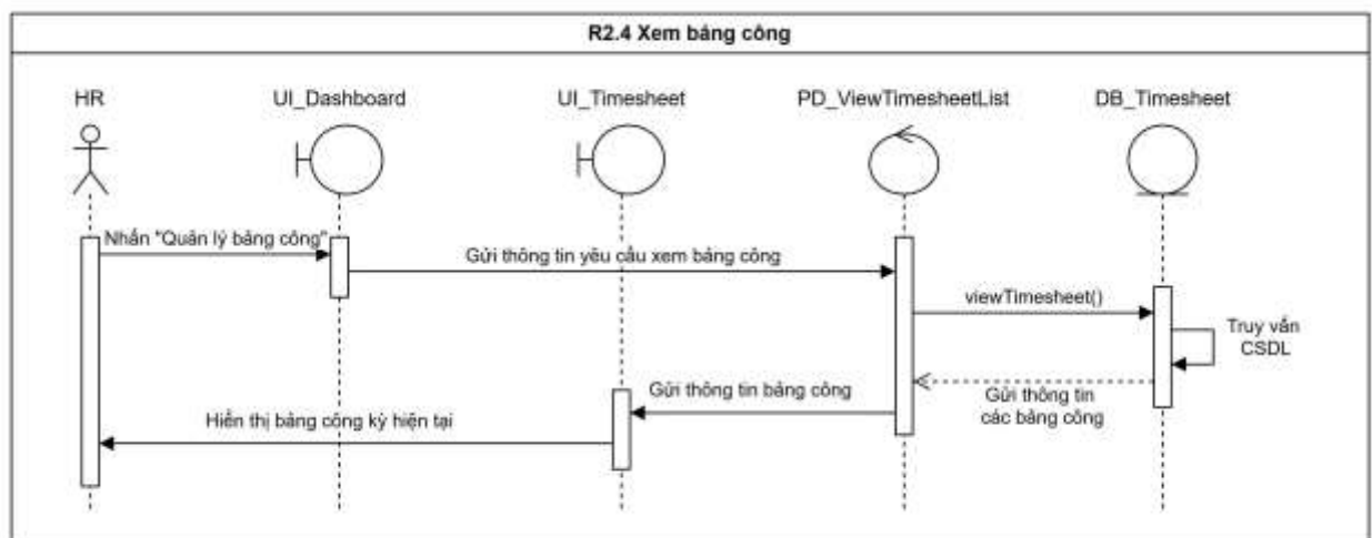
Hình 3.16 Biểu đồ tuần tự “Xem danh sách bảng công”
