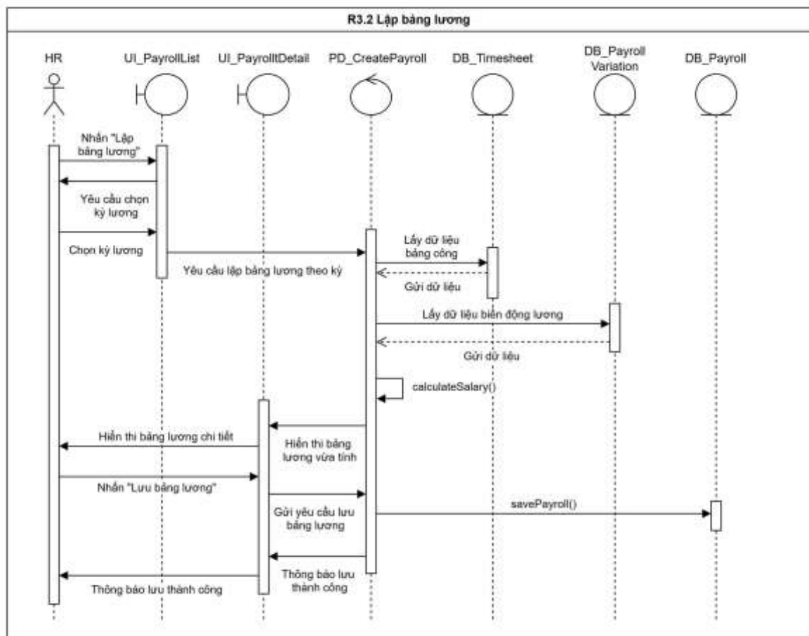
Hình 3.20 Biểu đồ tuần tự “Lập bảng lương tự động”
