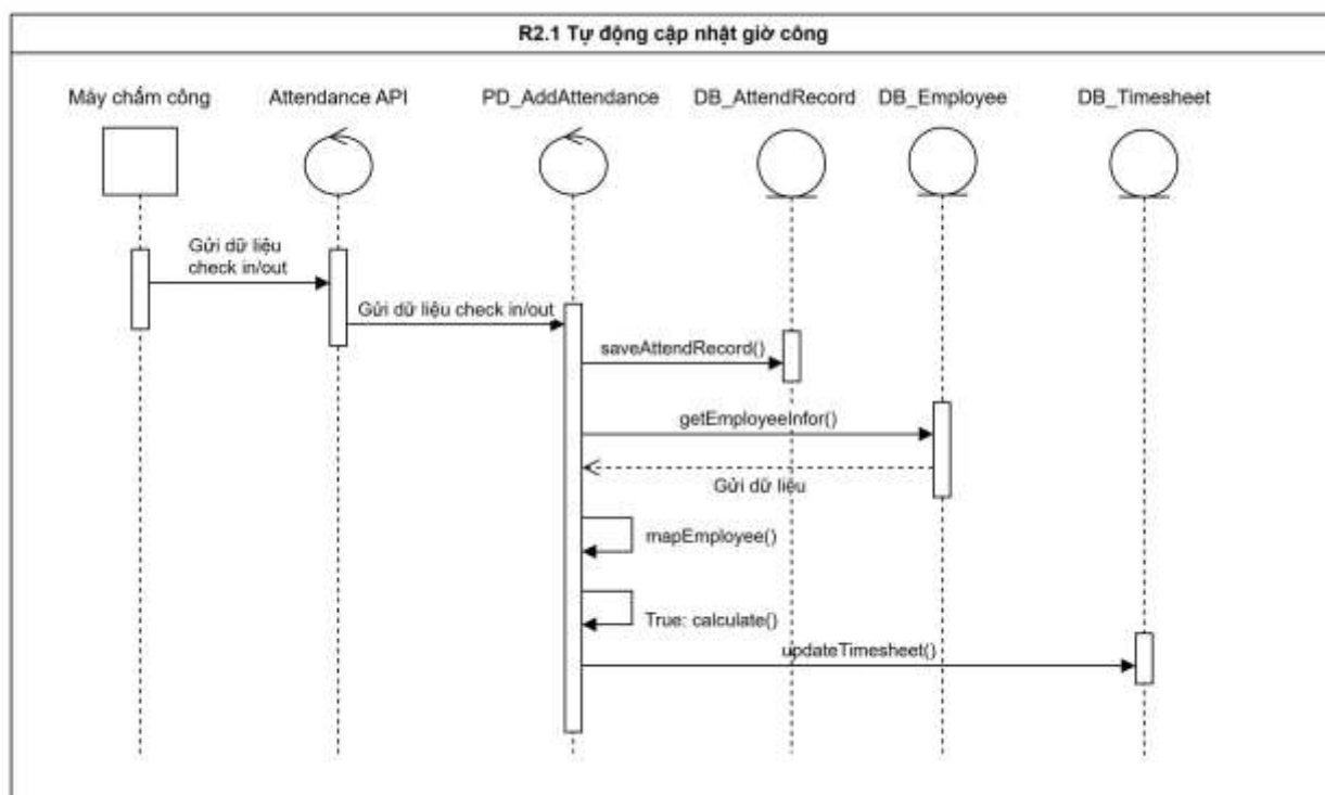
Hình 3.13 Biểu đồ tuần tự “Tự động cập nhật giờ công”
