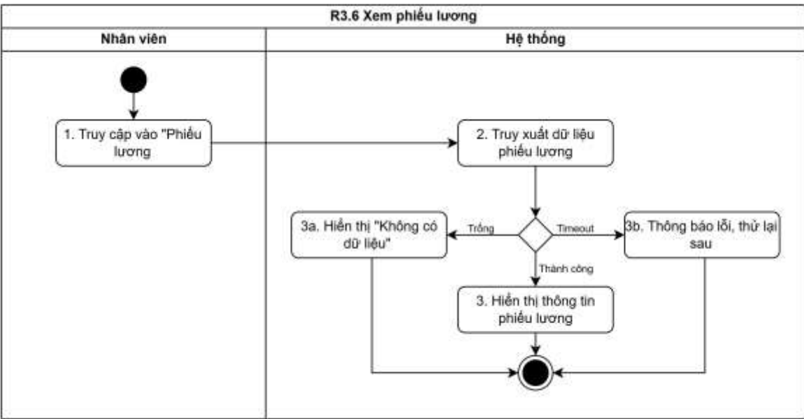
Hình 3.44 Biểu đồ hoạt động “Xem phiếu lương”
