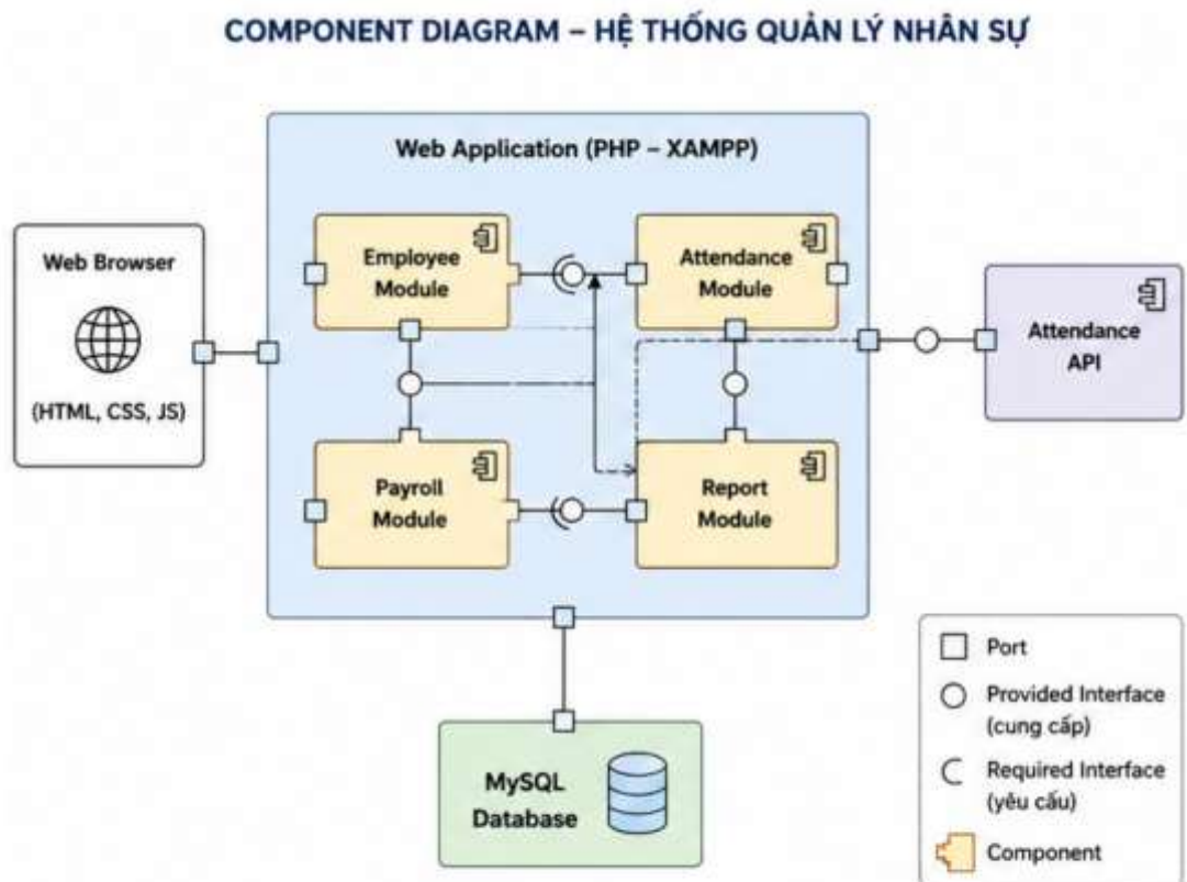
Hình 3.48 Biểu đồ thành phần
