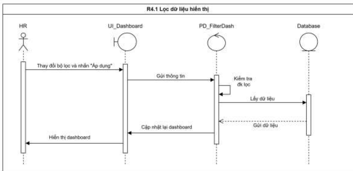
Hình 3.25 Biểu đồ tuần tự “Lọc dữ liệu hiển thị”
