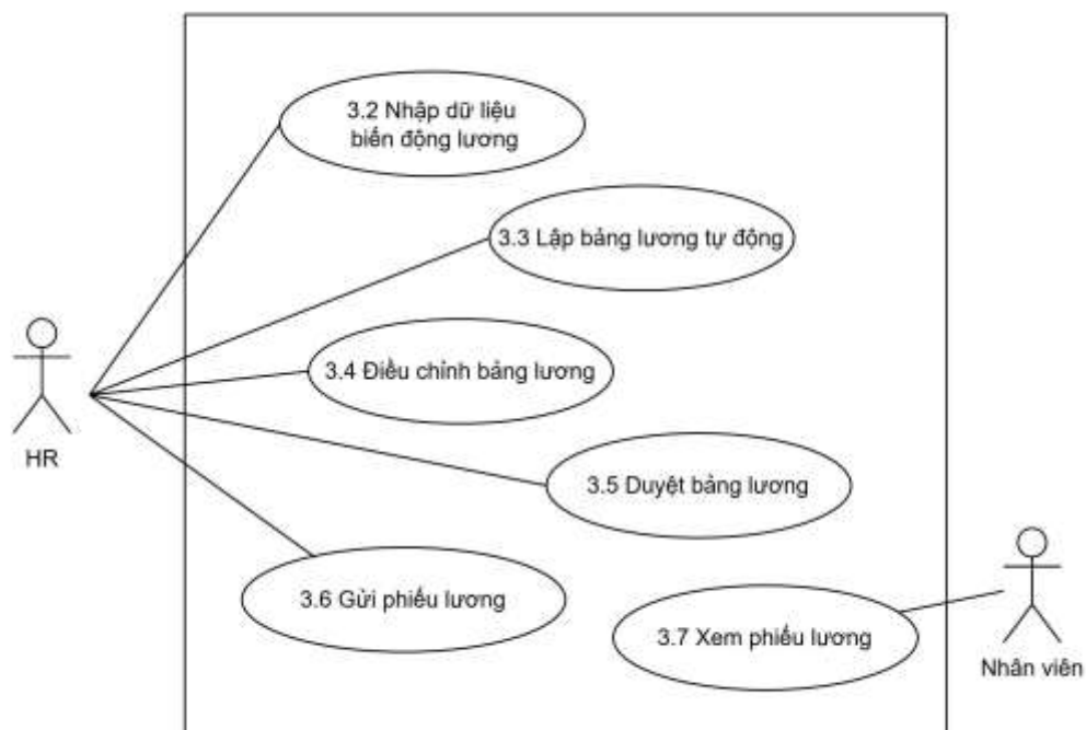
Hình 3.4 Biểu đồ Use Case Quản lý tiền lương
