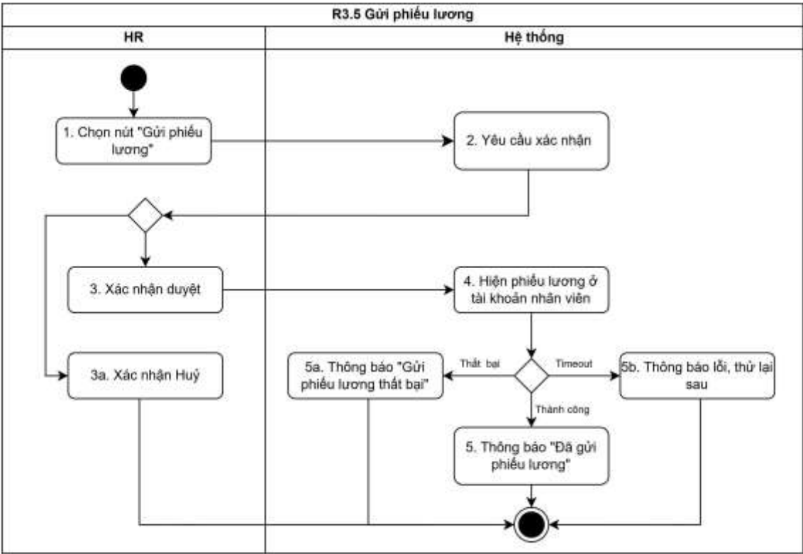
Hình 3.43 Biểu đồ hoạt động “Gửi phiếu lương”
