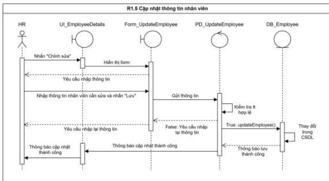
Hình 3.11 Biểu đồ tuần tự “Cập nhật thông tin nhân viên”
