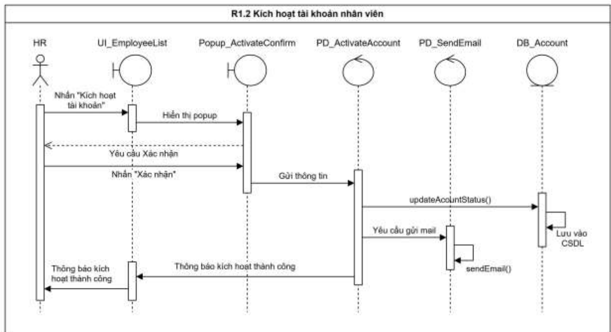
Hình 3.8 Biểu đồ tuần tự “Kích hoạt tài khoản nhân viên”
