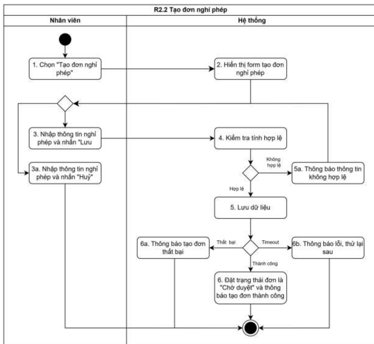
Hình 3.34 Biểu đồ hoạt động “Tạo đơn nghỉ phép”
