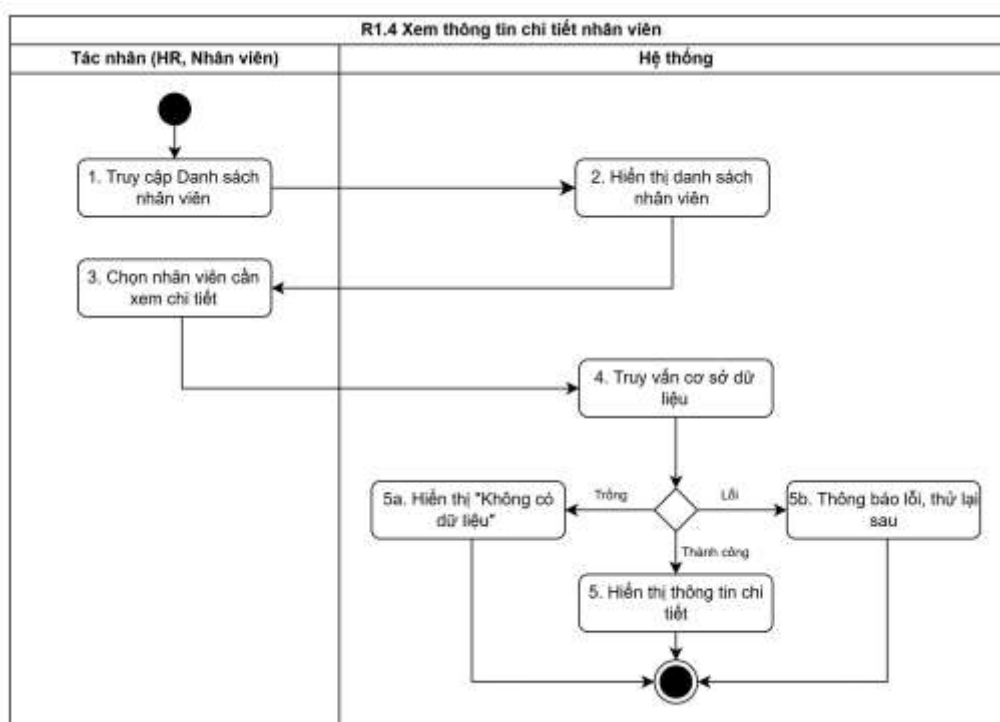
Hình 3.30 Biểu đồ hoạt động “Xem thông tin chi tiết nhân viên”
