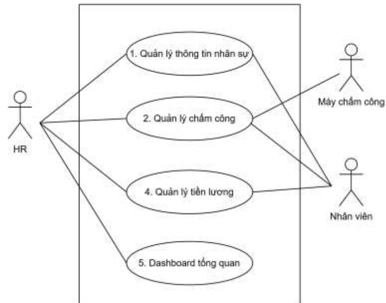
Hình 3.1 Biểu đồ Use Case tổng quát
