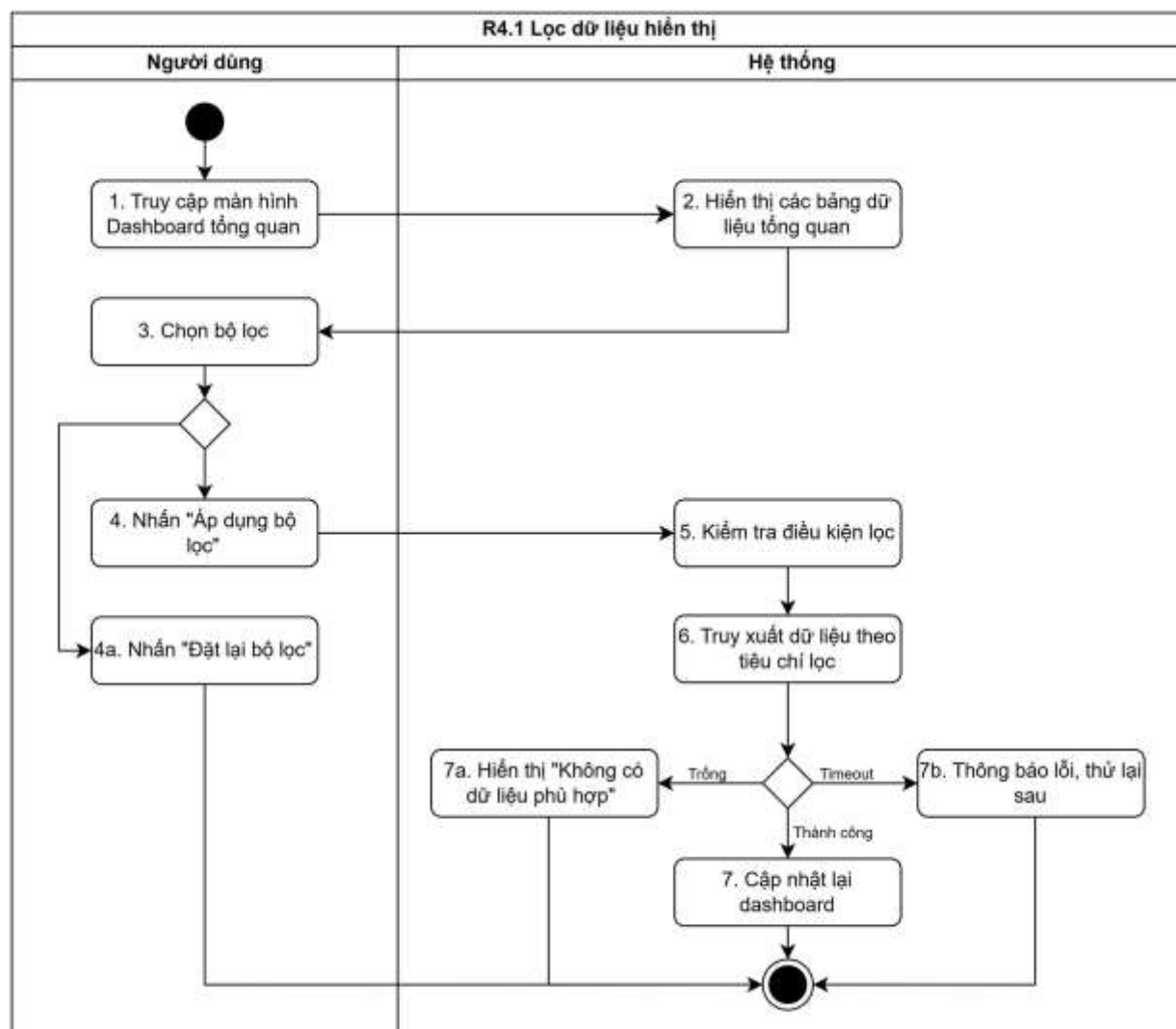
Hình 3.45 Biểu đồ hoạt động “Lọc dữ liệu hiển thị”
