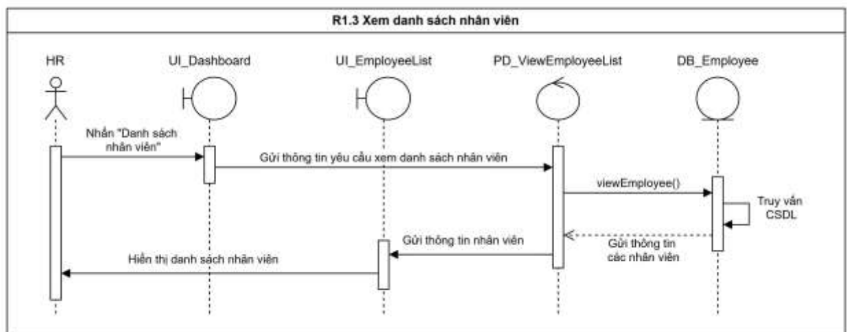
Hình 3.9 Biểu đồ tuần tự “Xem danh sách nhân viên”
