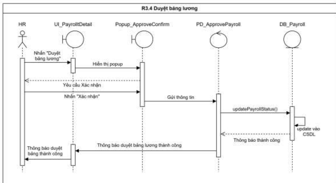
Hình 3.22 Biểu đồ tuần tự “Duyệt bảng lương”
