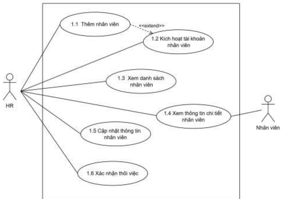
Hình 3.2 Biểu đồ Use Case Quản lý thông tin nhân sự
