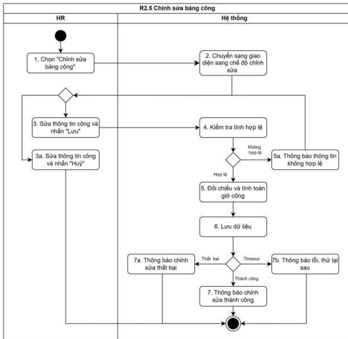
Hình 3.36 Biểu đồ hoạt động “Chỉnh sửa công”
