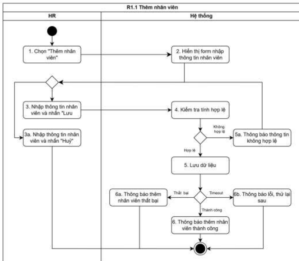
Hình 3.27 Biểu đồ hoạt động “Thêm nhân viên”
