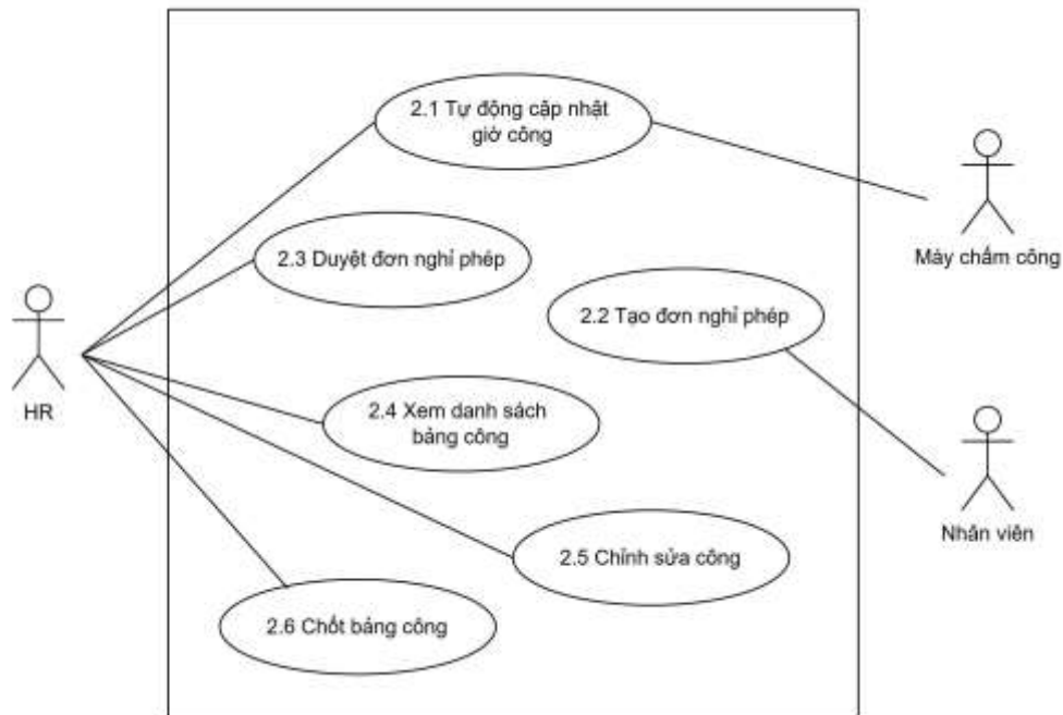
Hình 3.3 Biểu đồ Use Case Quản lý chấm công
