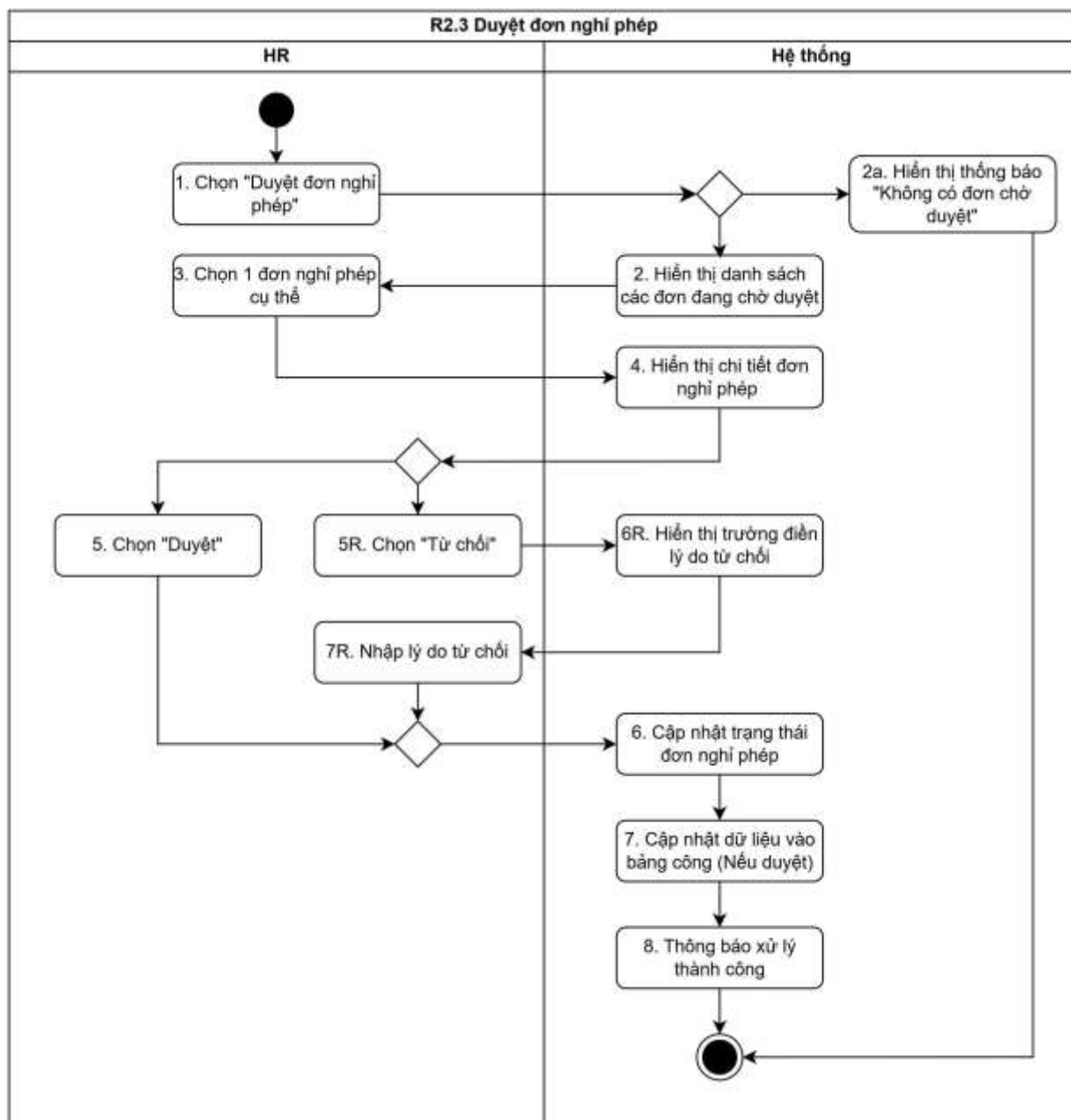
Hình 3.35 Biểu đồ hoạt động “Duyệt đơn nghỉ phép”
