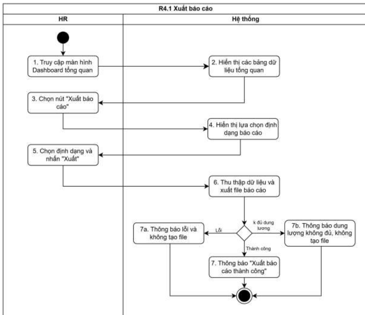
Hình 3.46 Biểu đồ hoạt động “Xuất báo cáo”
